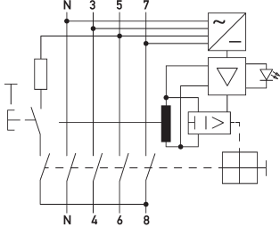
Anschlussschema
