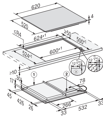
1) vorn, 2) Netzanschlusskasten mit Netzanschlussleitung, L = 1440 mm, wird dem Gerät lose beigelegt, 3) Stufenfräsung Natursteinarbeitsplatte, 4) Holzleiste 12 mm (kein mitgeliefertes Zubehör)
