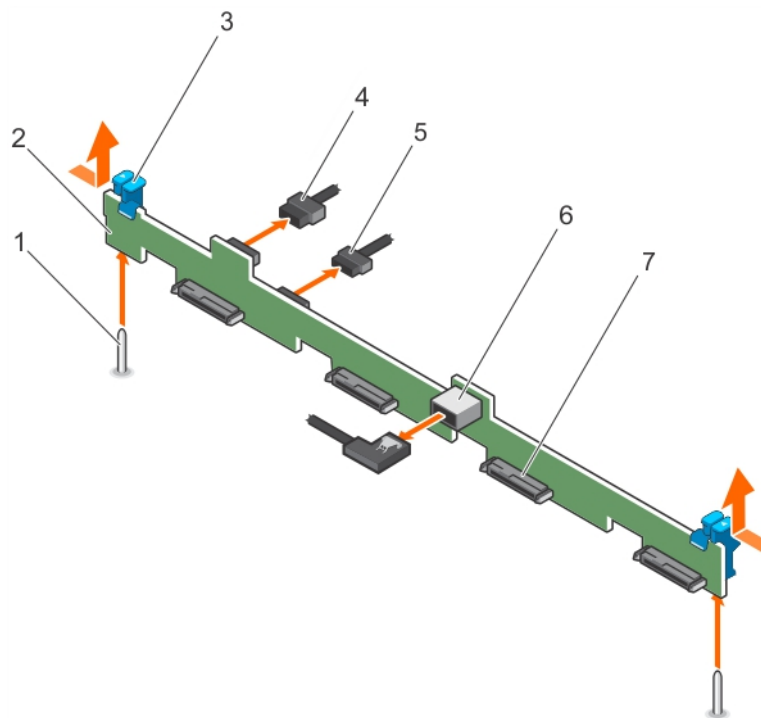
Abbildung 79. Entfernen der Rückwandplatine für vier 3,5-Zoll-SAS/SATA-Festplatten
