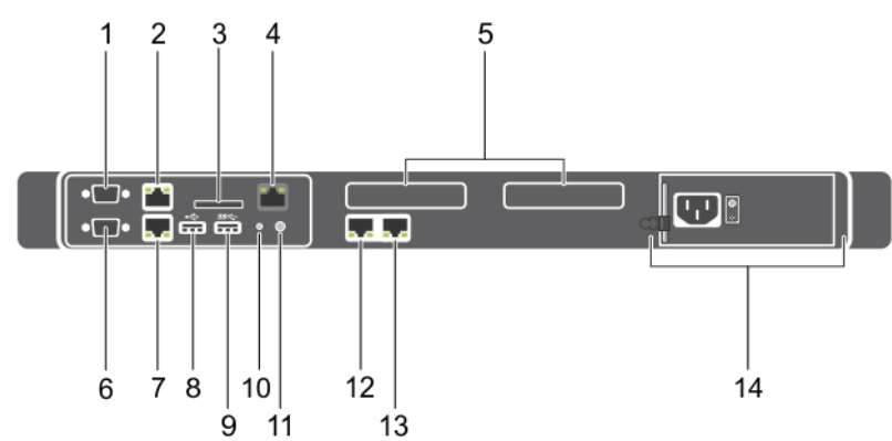
Abbildung 8. Funktionen auf der Rückseite – verkabeltes Netzteil
