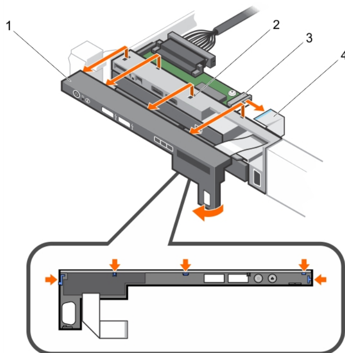
Abbildung 89. Entfernen des Bedienfelds – Gehäuse für acht 2,5 Zoll-Festplatten-/SSD-Laufwerke
