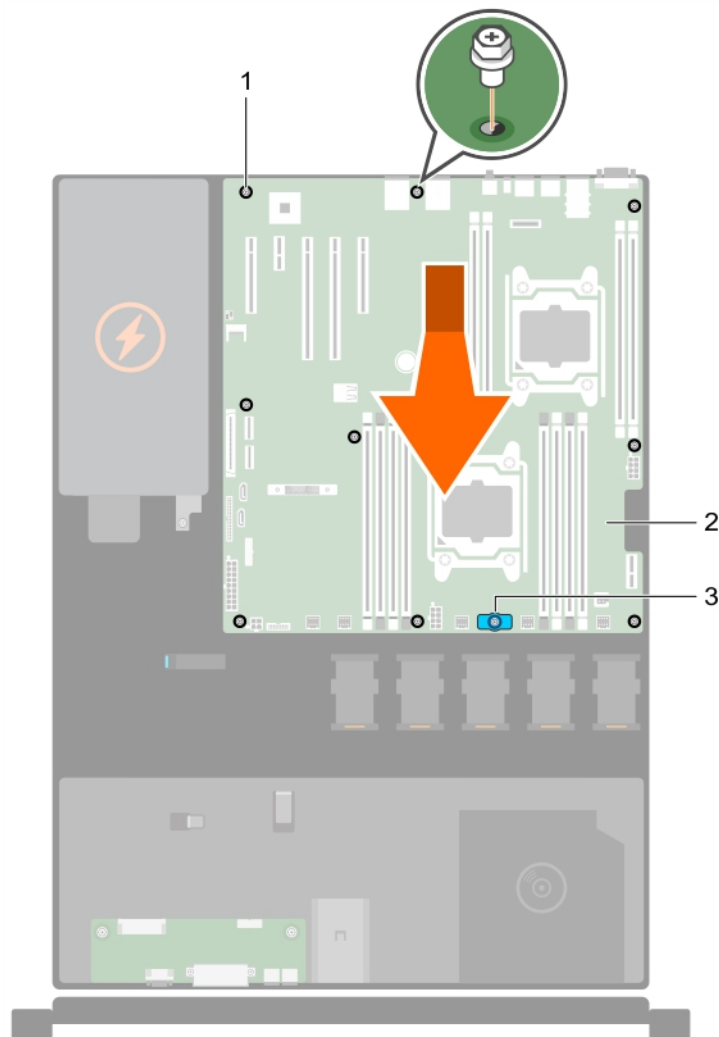
Abbildung 99. Einsetzen der Systemplatine
