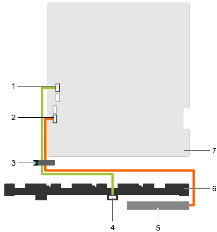
Abbildung 80. Verkabelungsschema – SAS/SATA-Rückwandplatine für vier 3,5-Zoll- oder 2,5-Zoll-Festplatten
