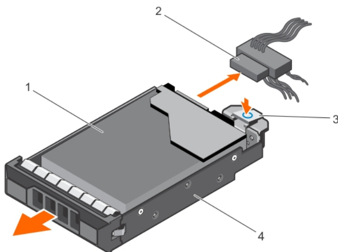
Abbildung 32. Entfernen eines Trägers für eine verkabelte Festplatte
