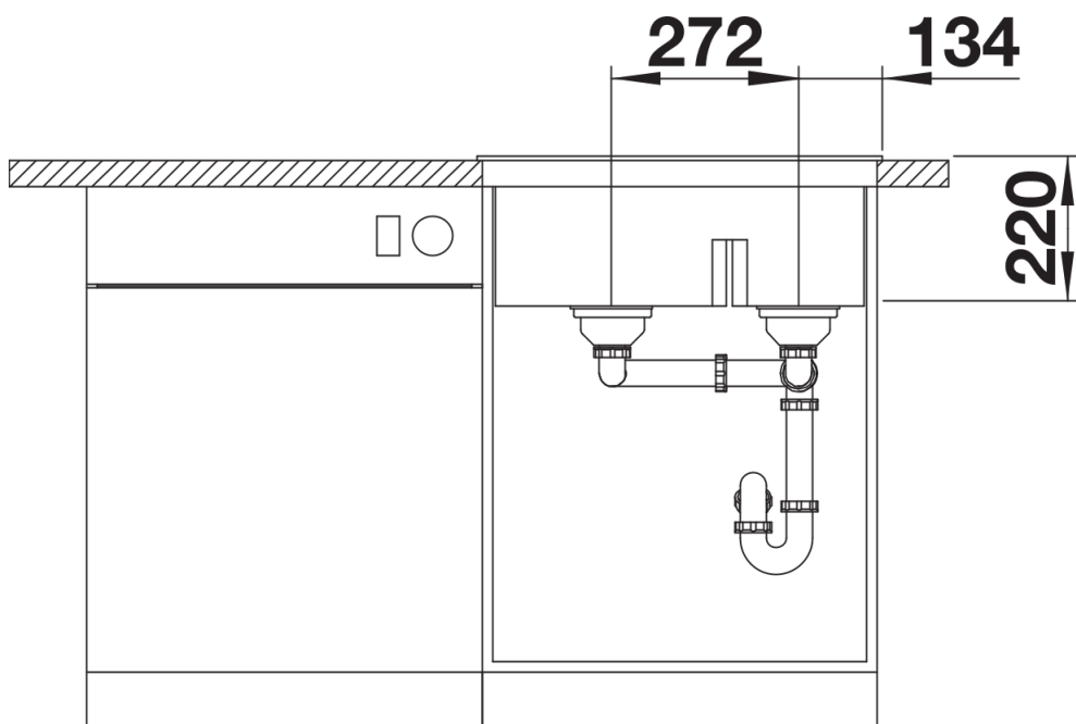
Frontansicht
