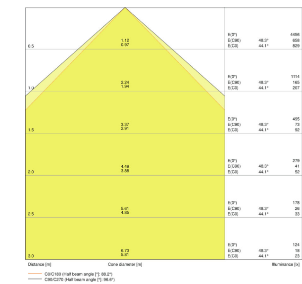
LVK Kegel
