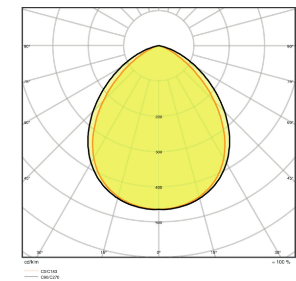
LVK Polar
