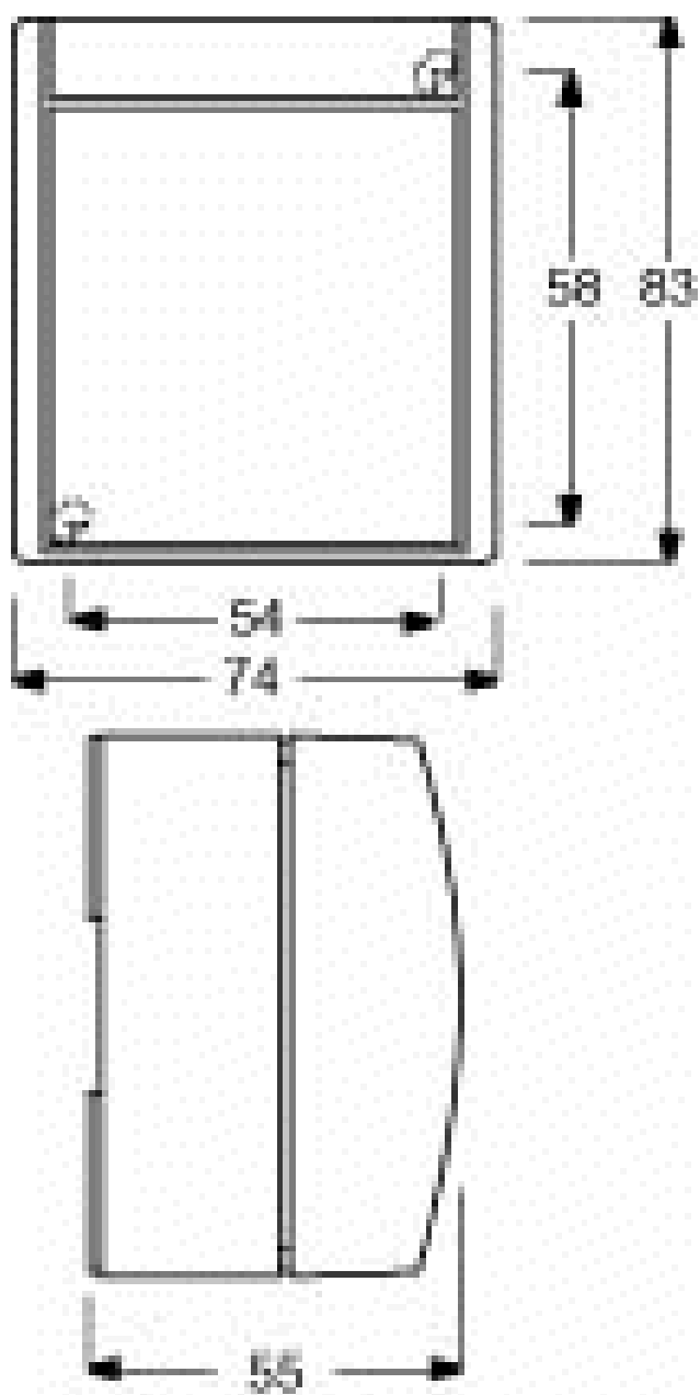
ocean® 1-fach Gehäuse mit Bohrmaßen
