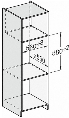
ESW7x20, Skizze
