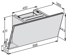
DAH2960EXTA Skizze
