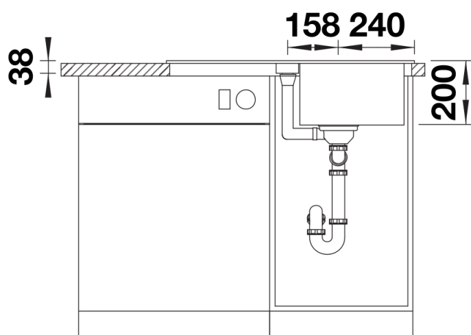
Frontansicht
