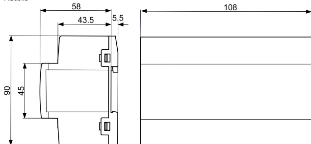
Maßbild
