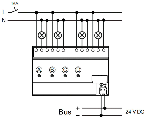
Anschlussbild
