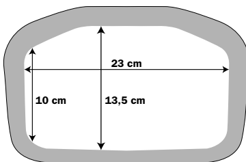
Abmessungen transparentes Deckelfach
