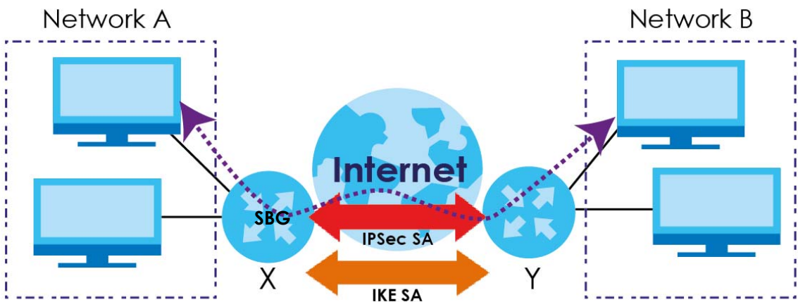
Figure 129 VPN: IKE SA and IPsec SA
