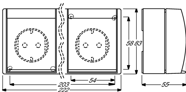
ocean® 3-fach waagerecht SCHUKO® Steckdosen mit Bohrmaßen
