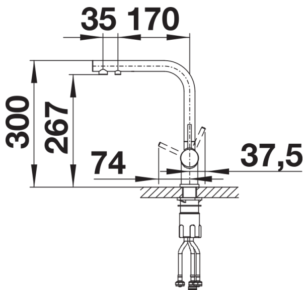
Seitenansicht
