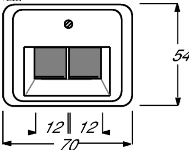
Maßbild
