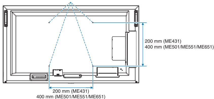
VESA-Montageadapter M6 (ME431/ME501/ME551), M8 (ME651)
