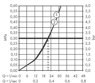
Durchflussdiagramm
