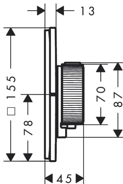
Maßzeichnung
