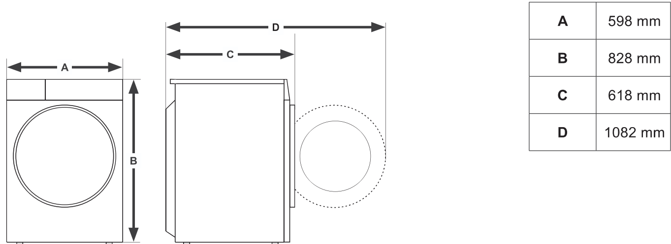
Abb. 5 Abmessungen
