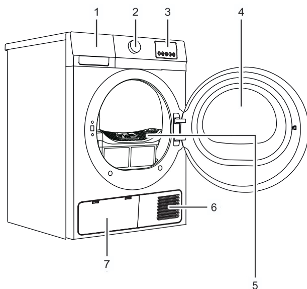
Abb. 2 Wäschetrockner WT8W1E, Vorderseite
