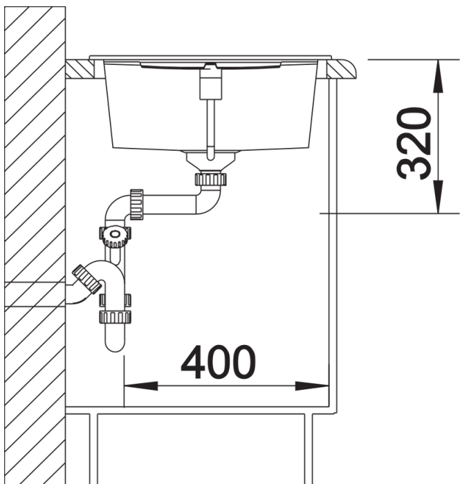
Seitenansicht
