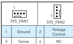
電壓模式風扇電源接頭
