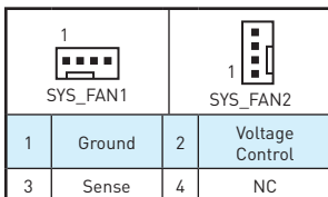
电压模式风扇接口
