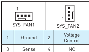
전압 모드 팬 커넥터
