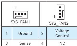
Lüfteranschluss des Spannung-Modus
