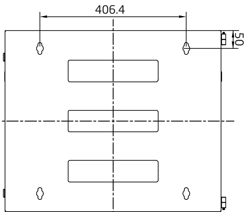
Hinteransicht
