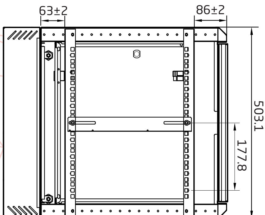
Seiteninnenansicht
