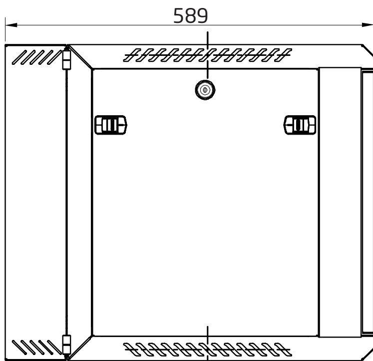
Seiteninnenansicht
