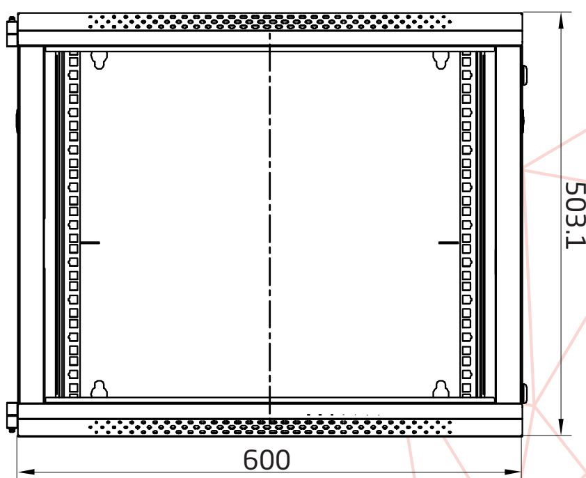
Vorderseiteninnenansicht
