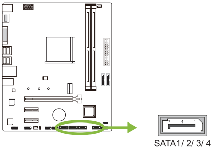
SATA1/ 2/ 3/ 4
