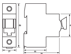
Maßzeichnung Gruppenansicht
