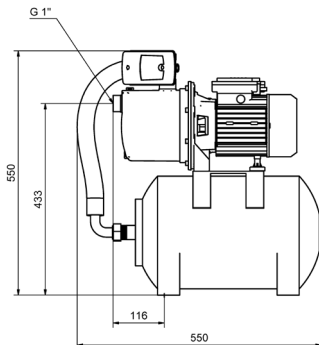
GARDEN 2000 mit ZPC 01 und Membranausdehnungsgefäß aus Edelstahl
