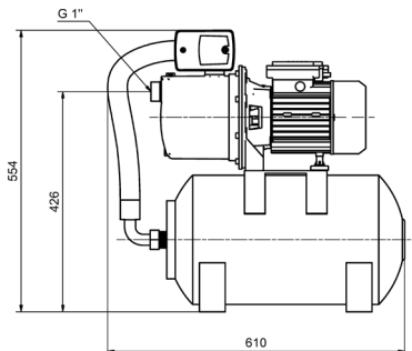
GARDEN 2000 mit ZPC 01 und Membranausdehnungsgefäß aus Stahl
