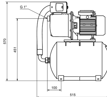
GARDEN 2000 mit ZPC 01 und Ausdehnungsgefäß aus Stahl mit Butylmembran
