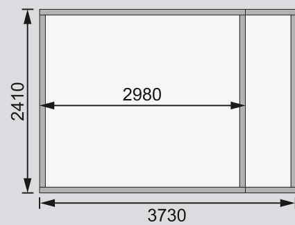
Fundamentplan ohne Boden (in mm)
