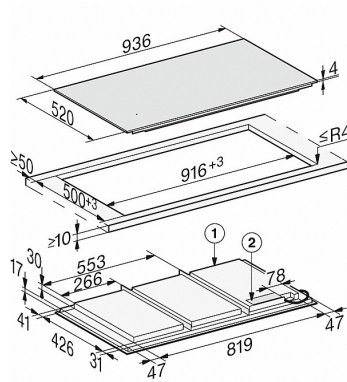
KM 7697 FL, KM 7897 FL (Skizze) aufliegend
