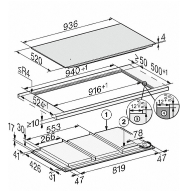
KM 7697 FL, KM 7897 FL (Skizze) flächenbündig
