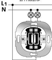
SCHÉMA DE RACCORDEMENT INTERRUPTEUR DOUBLE Δ I I IMAGE
