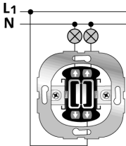
ANSCHLUSSSKIZZE SERIENSCHALTER
