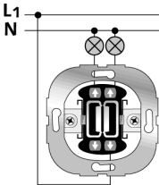
SCHEMA DI COLLEGAMENTO INTERRUTTORE IN SERIE
