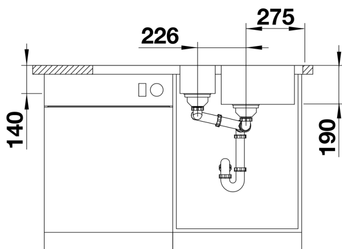
Frontansicht
