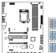
2x N/A + 1x M.2 SATA SSD Slot -- 5x SATA HDDs
